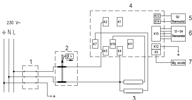
Електросхема
