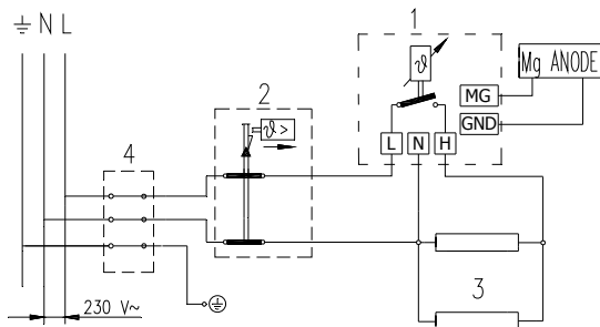
Электросхема
