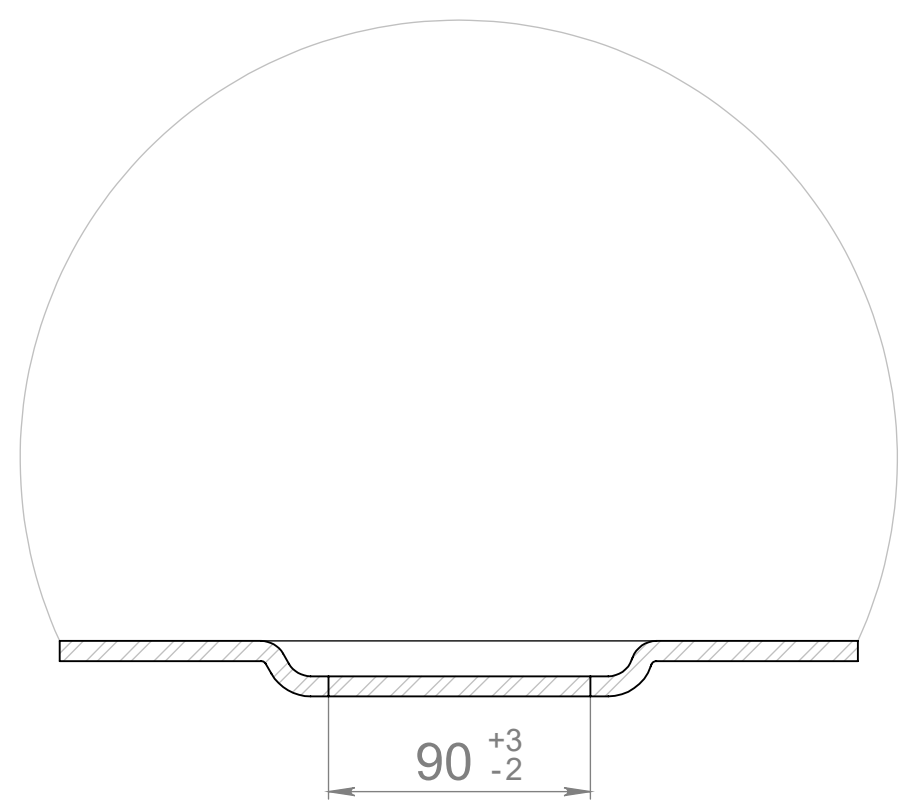
Сливное отверстие (вид сбоку)
