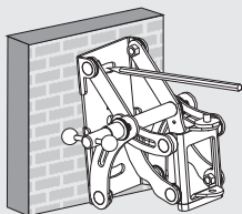
Монтаж к бетонной или кирпичной стене
