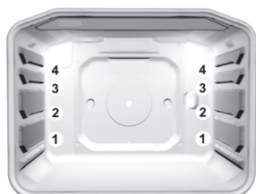
рельефные направляющие
