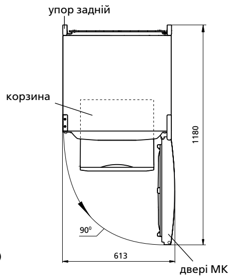
Рисунок 2 – Холодильник (вид зверху)
