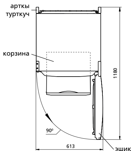
Сурот 2 – Муздаткыч (устунон корунушу)
