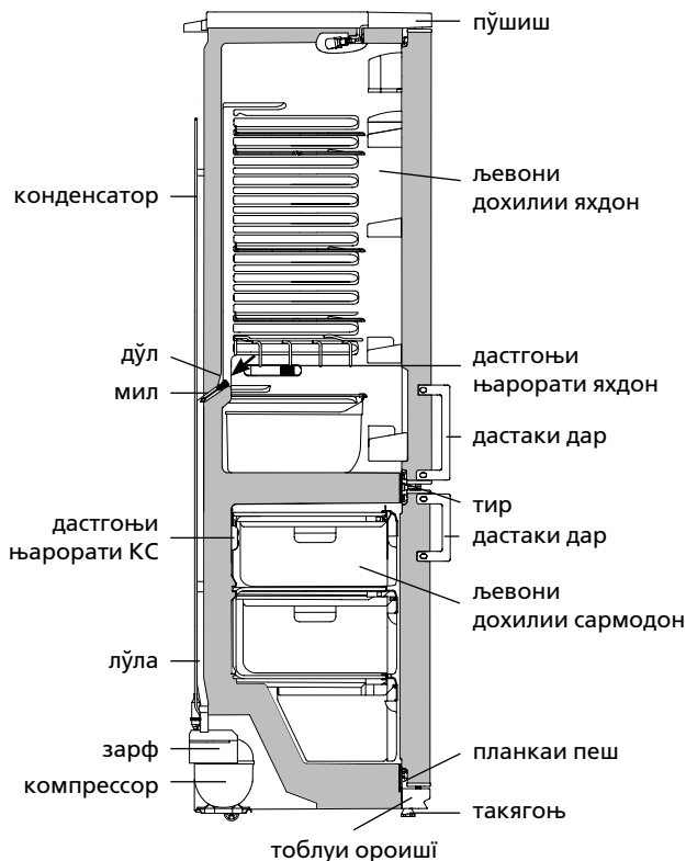
Расми 7 – Наќшаи партоби оби яхдон
