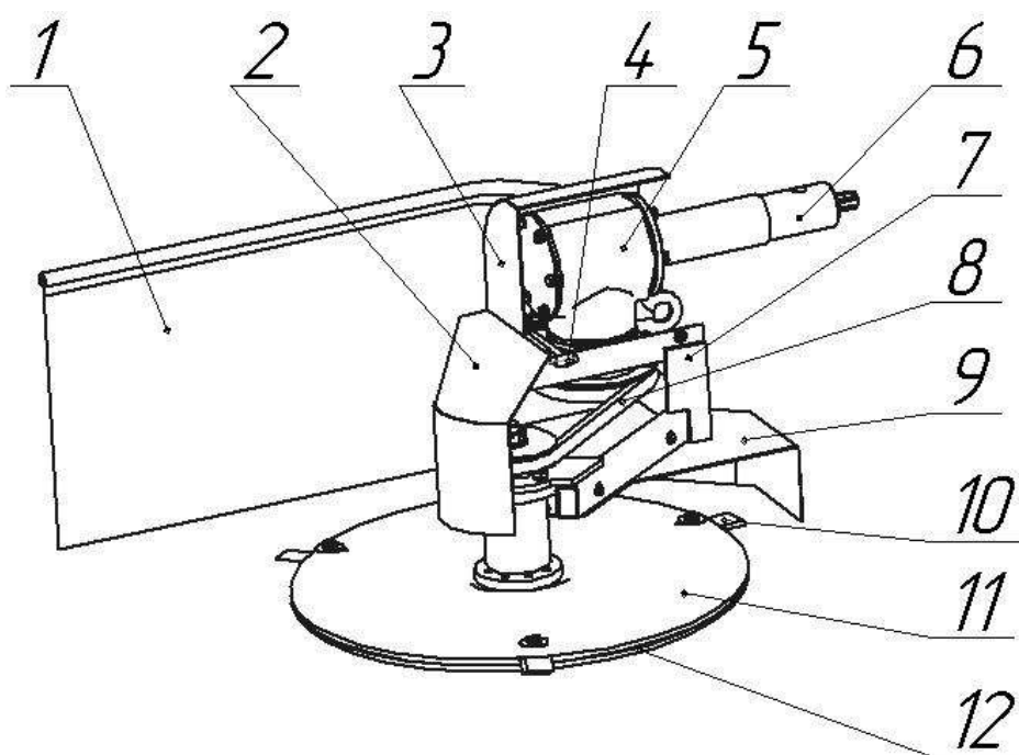
Рисунок 1 – Косилка роторная КРМ-1
