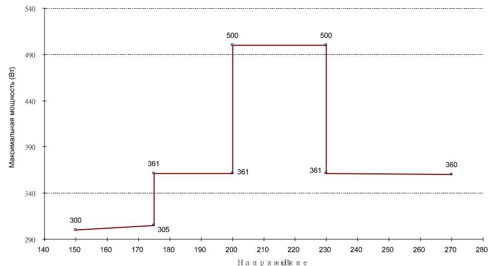
График зависимости максимальной мощности нагрузки от входного напряжения сети для iPOWER 1000
