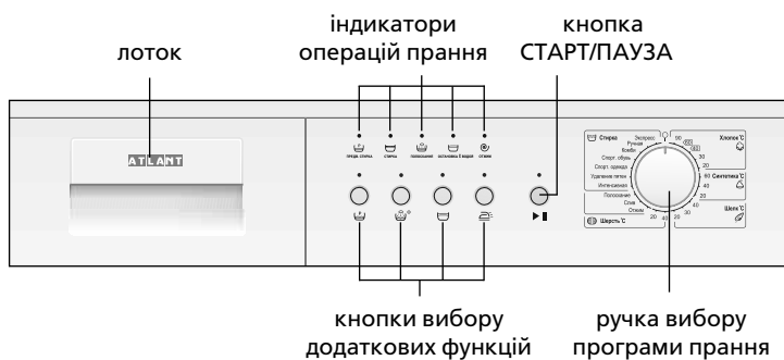
Рисуючи 1 – Панель керування
