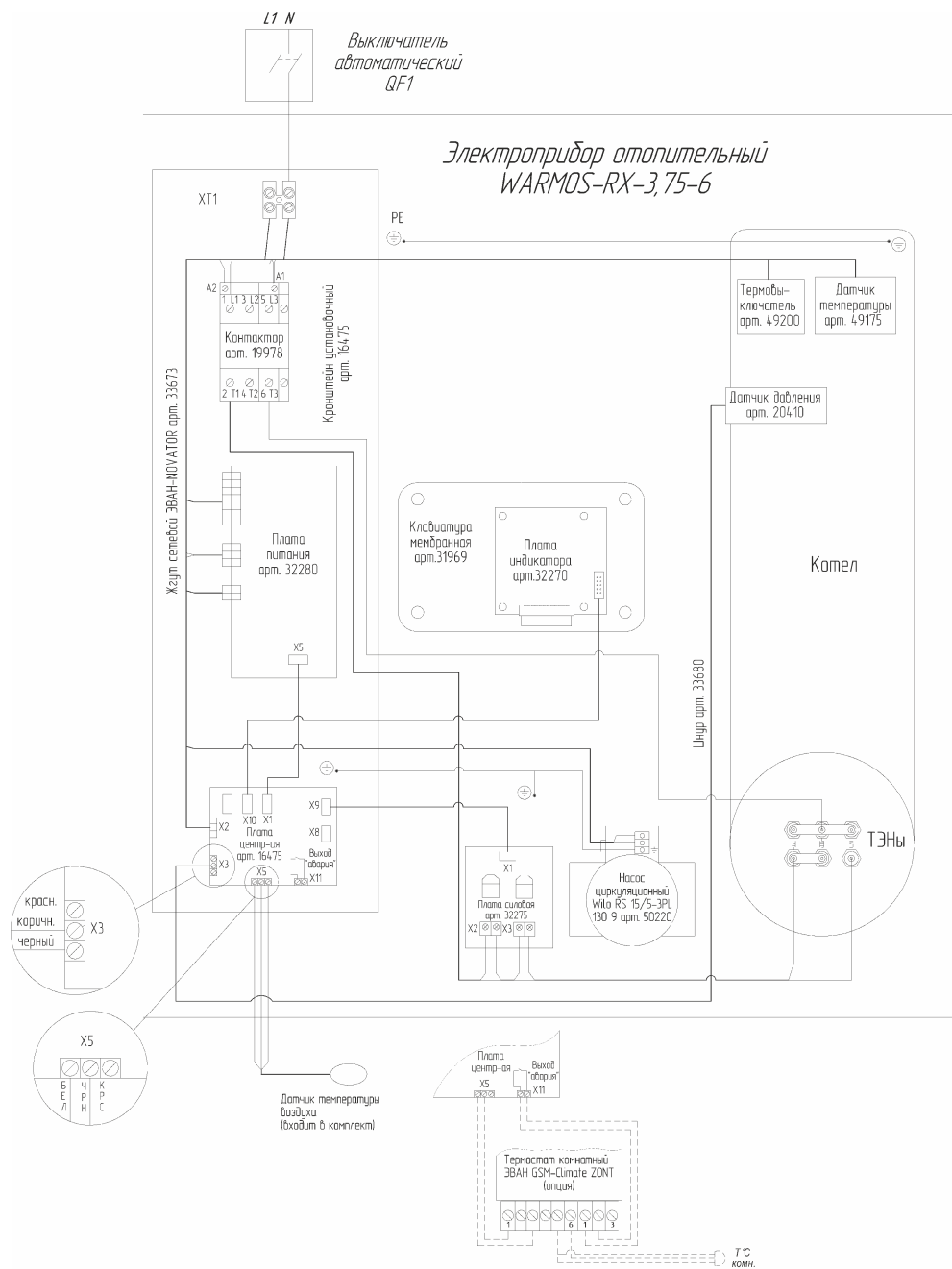
Рисунок 6 Схема подключения WARMOS-RX -3.75-6
