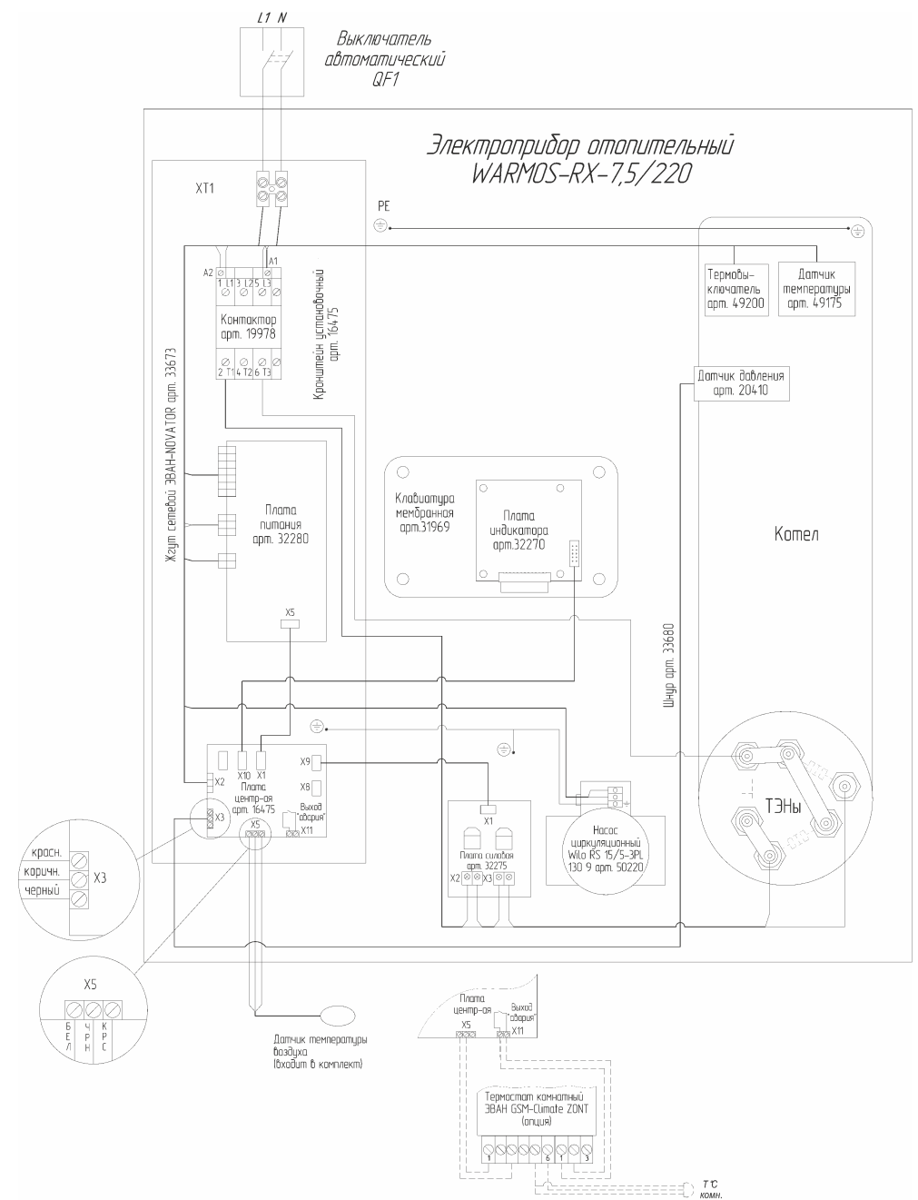
Рисунок 7 Схема подключения WARMOS-RX -7,5 (220 В)
