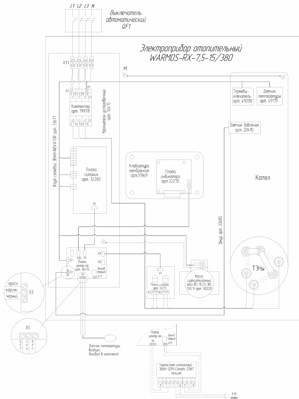
Рисунок 8 Схема подключения WARMOS-RX -7,5-15 (380)
