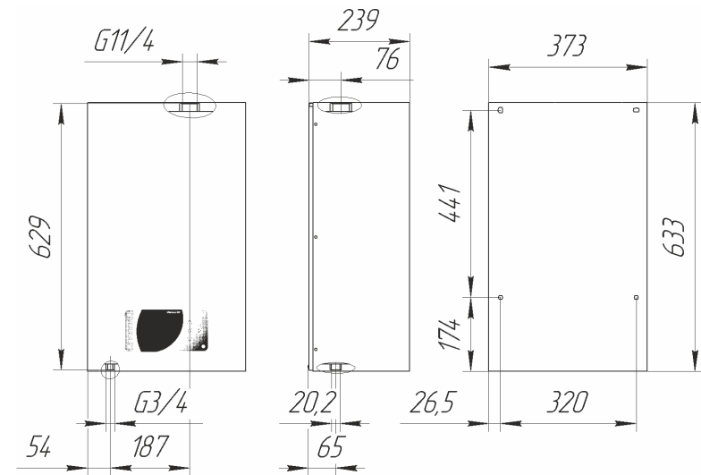
Рисунок 4. Габаритные и присоединительные размеры
