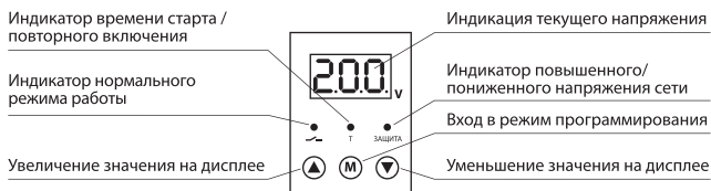
Рисунок 3. Лицевая панель реле RH 2
