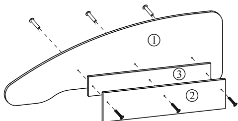
Сборка на левую сторону
