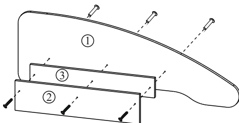
Сборка на правую сторону
