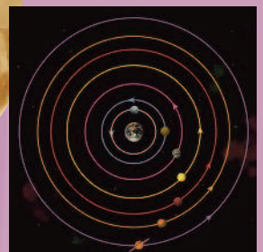
Система мира по Аристотелю и Птолемею
