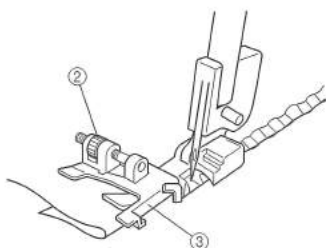
2 Stilleskrue 3 Føring
