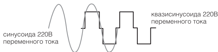
Сравнение квазисинусоиды и чистой синусоиды
