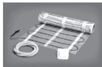
Комплект кабельной системы 1. Мат нагревательный 2. Терморегулятор 3. Трубка для термодатчика с заглушкой
