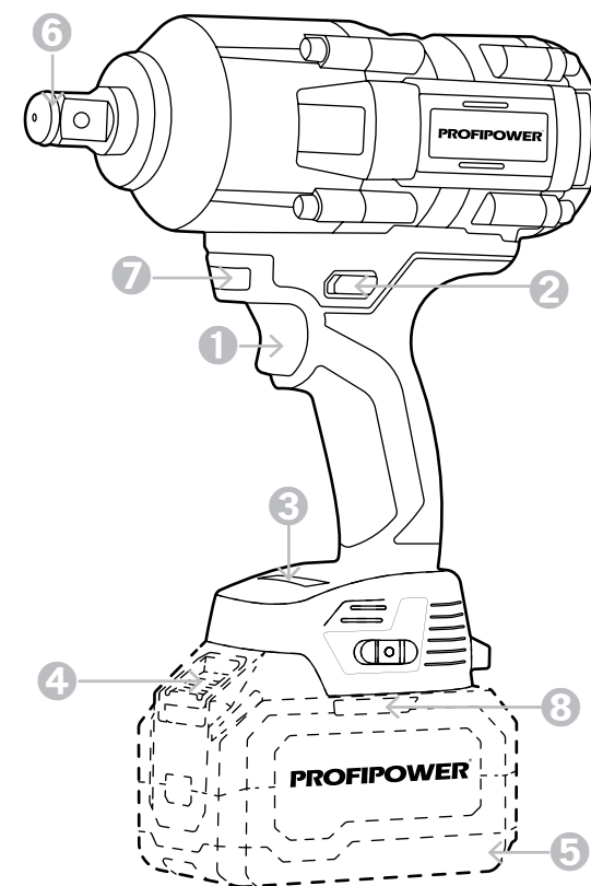
Рисунок 1.5. Устройство изделия
