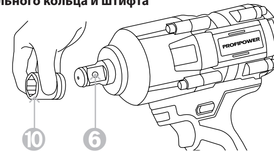
Рисунок 2.2.5.1. Установка ударной головки без уплотнительного кольца и штифта
