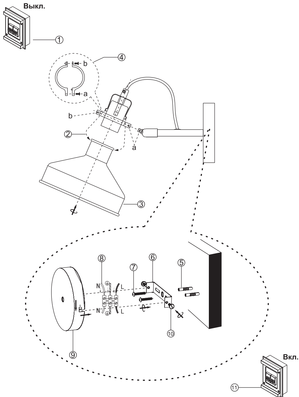
Рис.2 Сборка и установка светильника.
