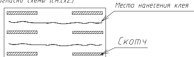
Схема нанесения клея на зеркало (Сх.2)
