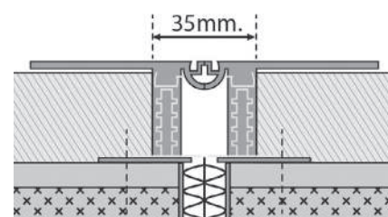
Рис. 22. MIGUA – заделка деформационных осадочных швов Fr30
