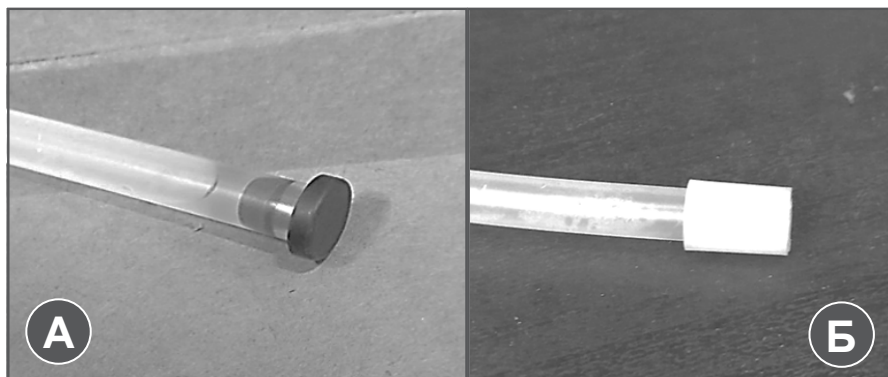
Рис. 3 Замена заглушки на фильтрующую сетку
