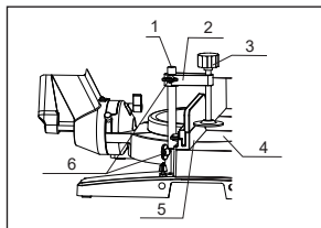
1. Шпindel 2. Держатель 3. Винт 4. Барашковый болт 5. Поворотное основание 6. Перегораживающая пластина
