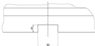
Эскиз А. Задний бампер.
