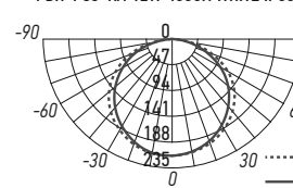
РВН-РС3-РА 12W 4000K WHITE IP65
