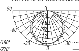
РВН-РС4-РА 12W 4000K CL P65
