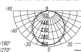
РВН-РС4-РА 10W 4000K CL IP65
