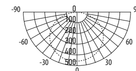
РВН-РС2-РА 18W
