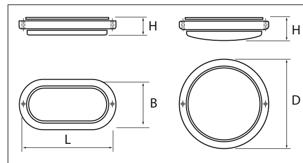
Габаритные размеры вентильников PBH-PC2
