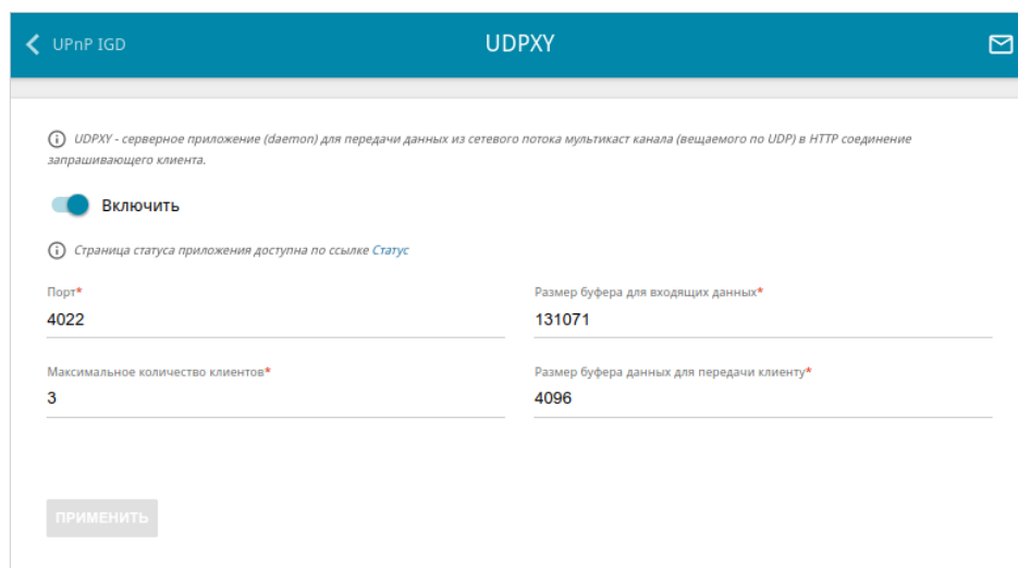
Рисунок 145. Страница Дополнительно / UDPXY .
