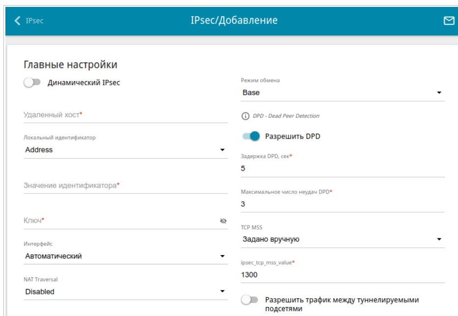
Рисунок 150. Страница добавления IPsec-туннеля. Раздел Главные настройки .
