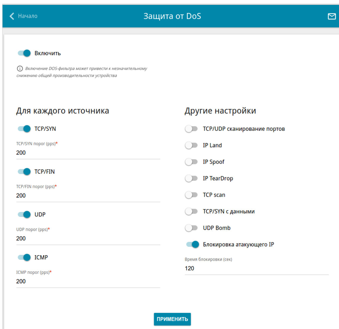
Рисунок 161. Страница Межсетевой экран / Защита от DoS .
