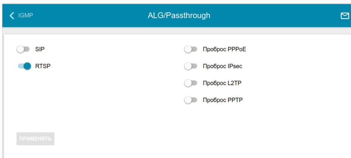
Рисунок 148. Страница Дополнительно / ALG/Passthrough .
