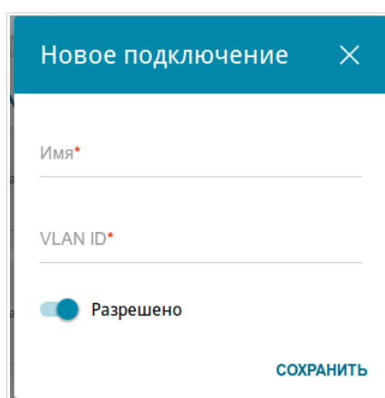
Рисунок 47. Добавление подключения.
