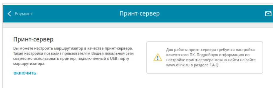
Рисунок 109. Страница Принт-сервер .
