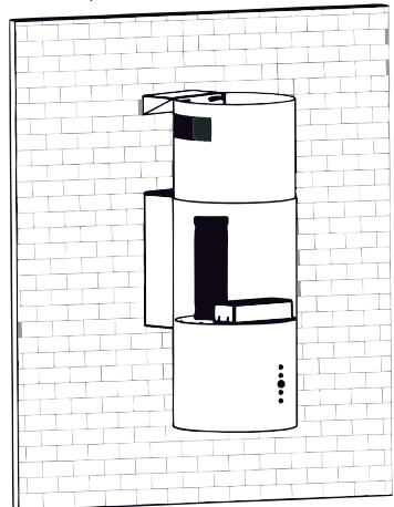
Рис. 8 Схема монтажа вытяжки
