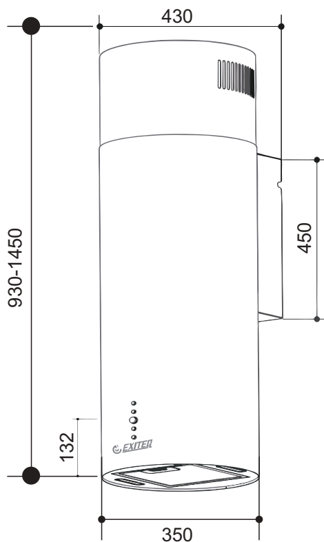
Рис. 1 Внешний вид кухонной вытяжки и схема размеров
