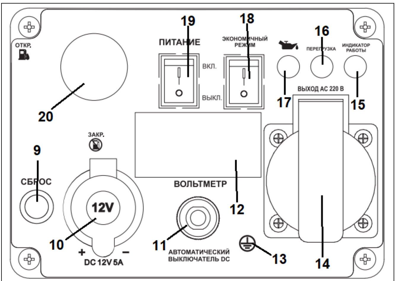
Рис. 2. Панель управления
