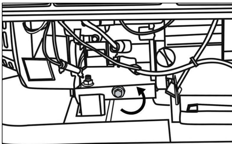
Рис. 10. Слив масла
