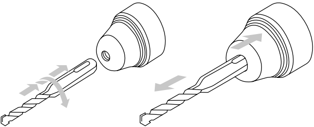
Рисунок 2.2.3. Установка оснастки Рисунок 2.2.3.1. Снятие оснастки
