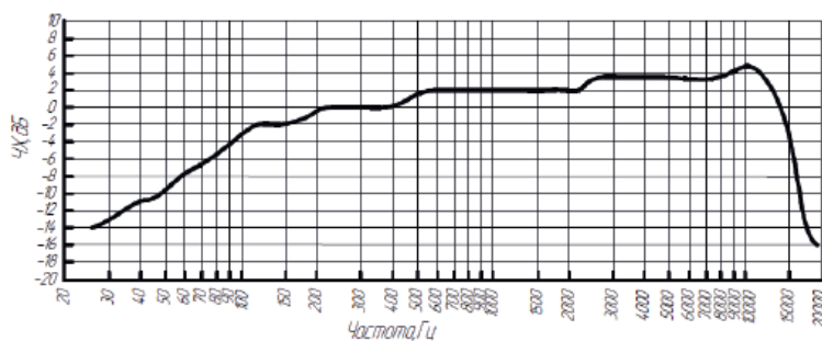
Амплитудно-частотная характеристика капсюля OWS-HC01.
