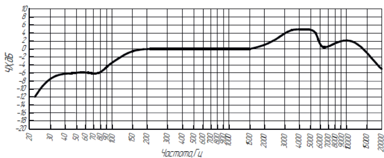
Амплитудно-частотная характеристика капсюля OWS-HC02.
