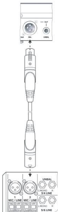
Схема подключения А
