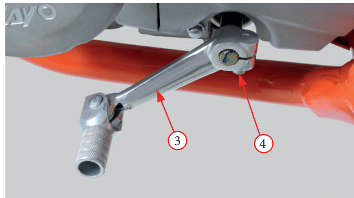
Фото 5.14. Регулировка положения рычага передач
