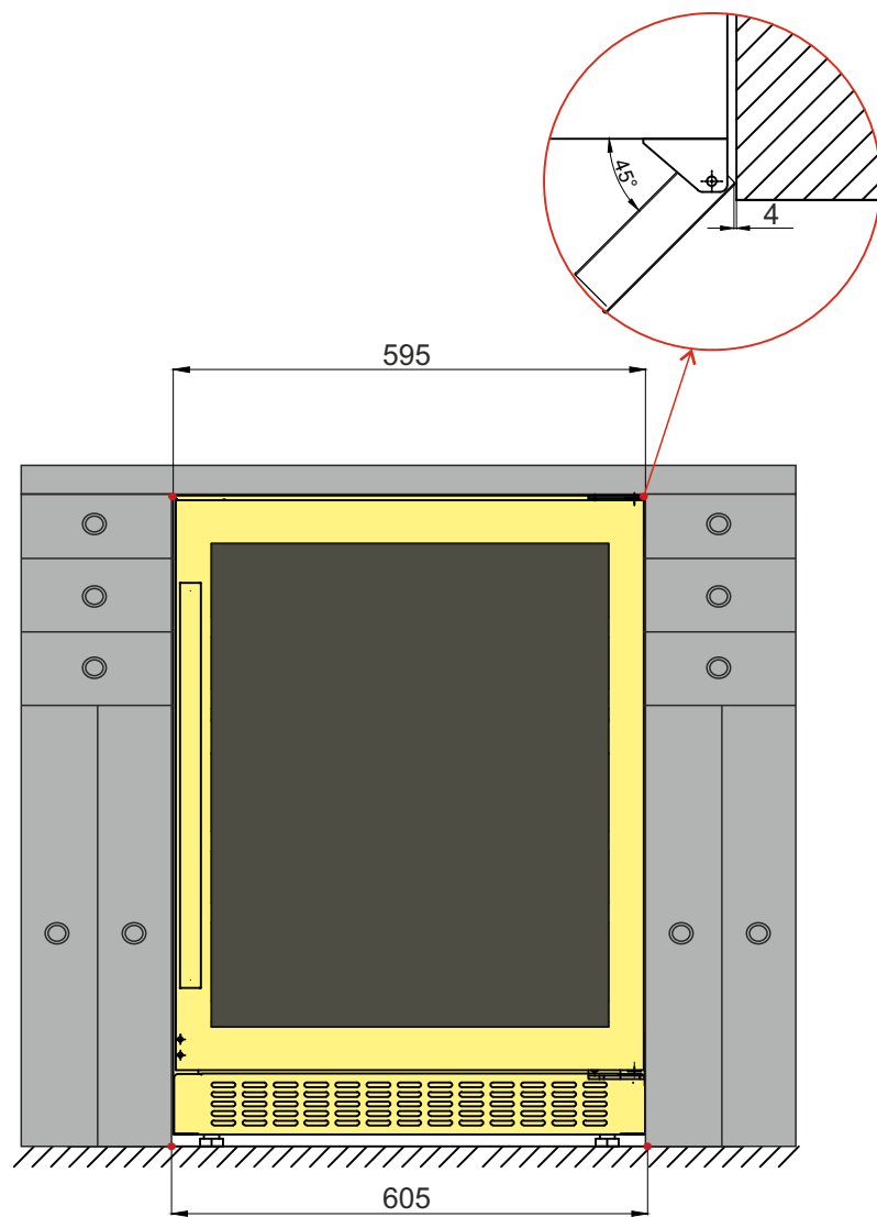
ВИД СПЕРЕДИ
