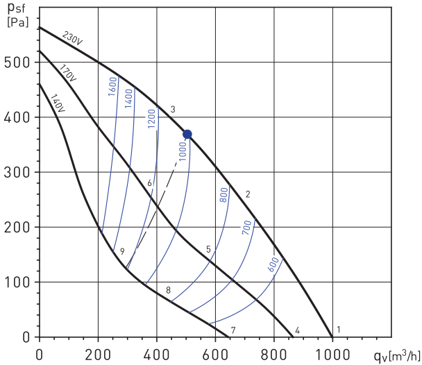
VENT /V-250N
