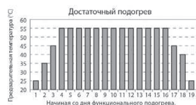
Рис. 16. Достаточный подогрев
