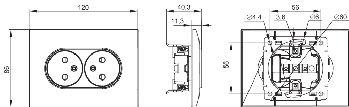
и) двухместная розетка без контактов заземления с рамкой пластик / double-gang socket without ground contacts with plastic frame / пластмасса жақтауымен жерге тұйықтау контактілері жоқ қос желілік розетка / prize duble de rețea fără contacte de împământare cu cadru din plastic
