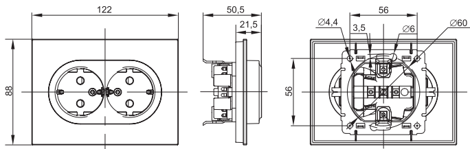
ж) двухместная розетка с контактами заземления с рамкой стекло/металл / double-gang socket with ground contacts with glass/metal frame / шыны/металл жақтауы бар жерге қосу контактілері бар қос розеткалар / prize duble de rețea cu contacte de împământare cu cadru sticlă/metal
