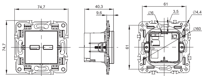
f) розетка / socket / prizele USB A+A
