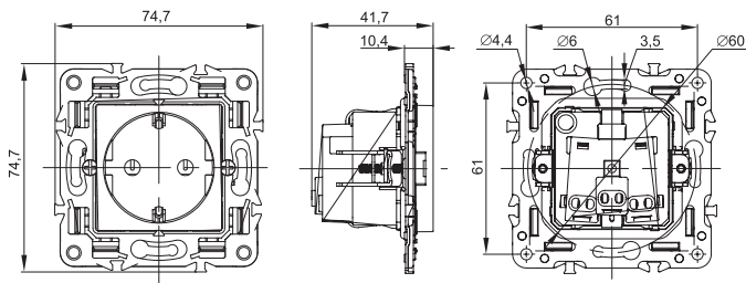
b) розетка с контактами заземления / socket with ground contacts / жерге тұйықтау түйіспелері бар розеткалар / prize cu contacte de împământare
