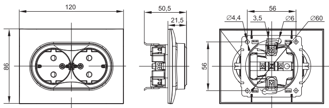
к) двухместная розетка с контактами заземления с рамкой пластик / double-gang socket with ground contacts with plastic frame / желілік қос розеткалар пластикалық жақтауы бар жерге тұйықтау контактілері / prize duble de rețea cu contacte de împământare cu cadru din plastic
