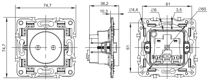
a) розетка без контактов заземления / socket without ground contacts / жерге тұйықтау түйіспелері жоқ розеткалар / prize fără contacte de împământare
