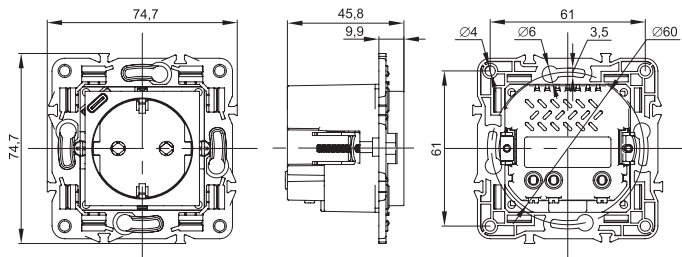
g) розетка с контактами заземления и USB – разъемом C / socket with ground contacts and USB-port C / жерге қосу контактілері мен C USB қосқыштары бар розетка / priză cu contacte de împământare și conectori usb C
