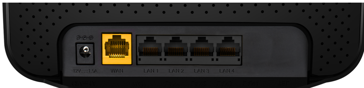
Рисунок 4. Вид задней панели DWR-953.
