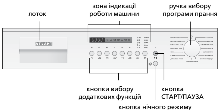
Рисунок 1 – Панель керування
