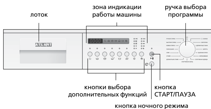
Рисунок 1 – Панель управления
